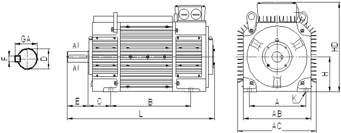
卧式、机座带底脚
