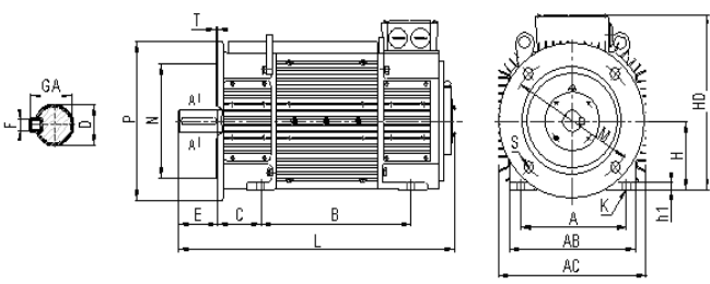
卧式、机座带底脚，端盖带凸缘
